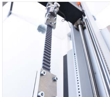
Zugversuch von Zahnriemen
